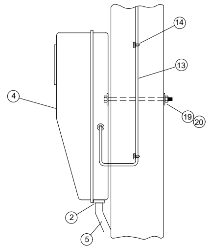
DETALLE MONTAJE CAJA DE EMPALME
